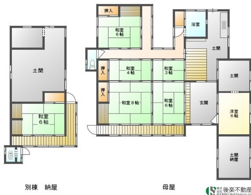
【間取り図】
