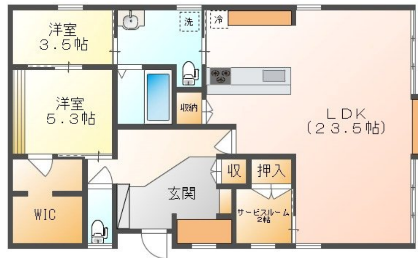
【間取り図】
